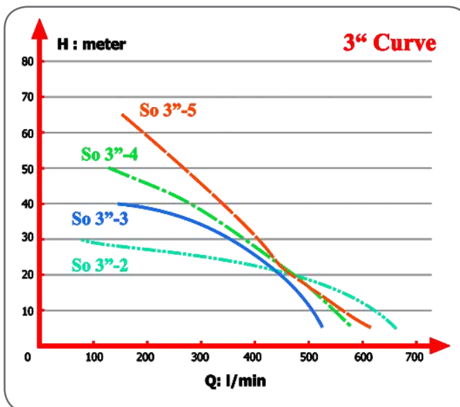
منحنی پمپ شناور اسپیکو مدل SO-3 اینچ
